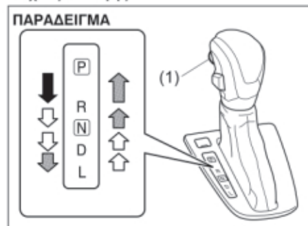
(1) Μπουτόν
